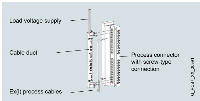
LK 393 cable guide
